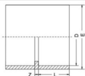
SOCKET
