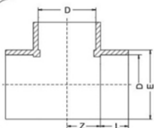
TEE 90°
